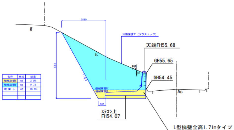
2-2' L型擁壁全高1.71mタイプ
